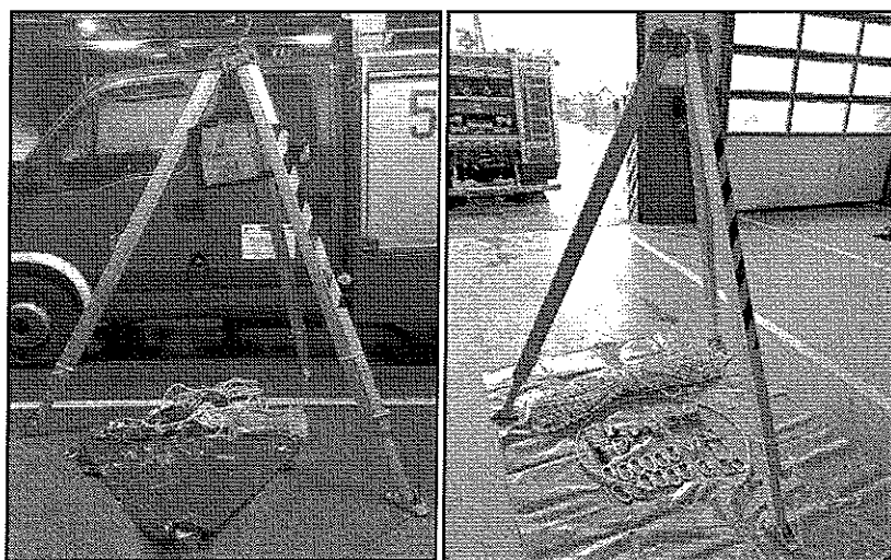
Zdjęcie 7. - Trójnóg ratowniczy z osprzętem
