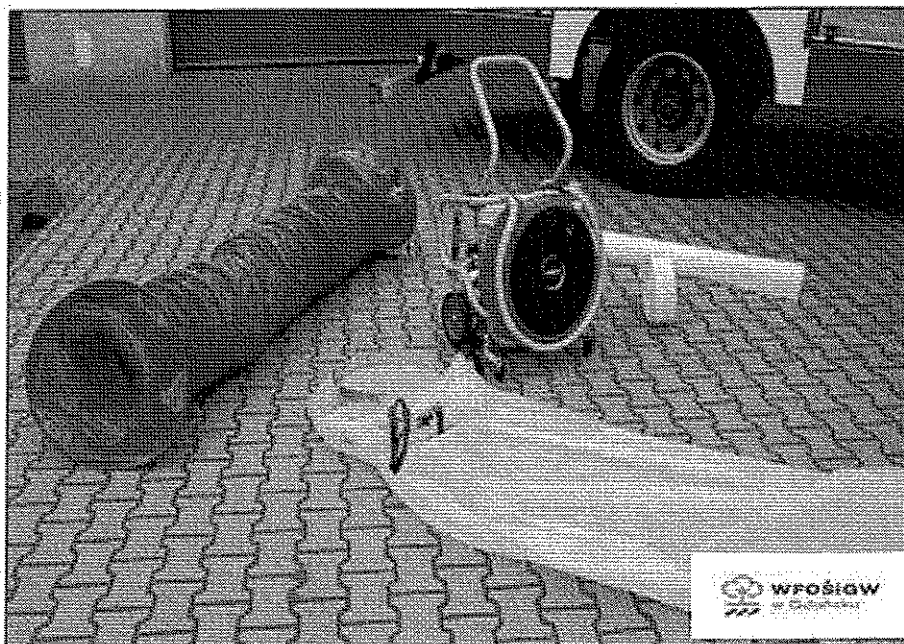
Zdjęcie 2. - Generator piany lekkiej
