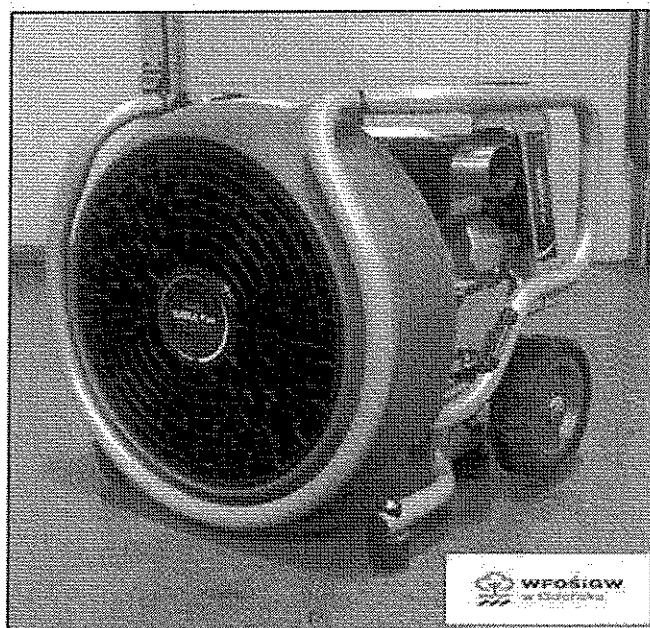
Zdjęcie 3. - Generator piany lekkiej z funkcją agregatu oddymiającego
