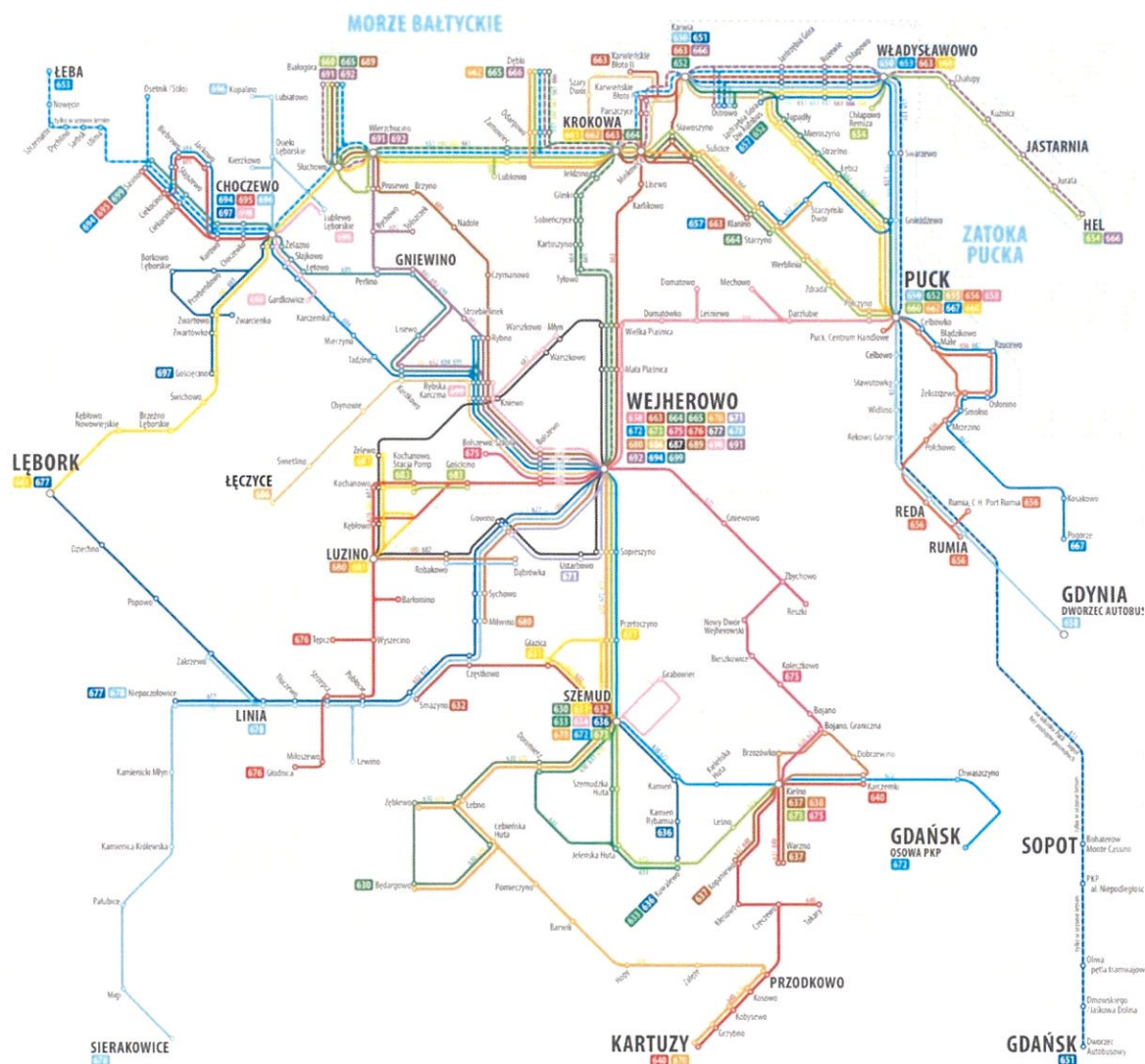
Rysunek 2 Schemat linii PKS Gdynia SA
